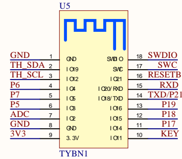
Bluetooth Module
