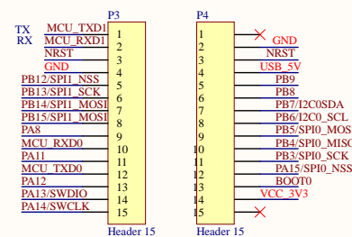
MCU管脚
