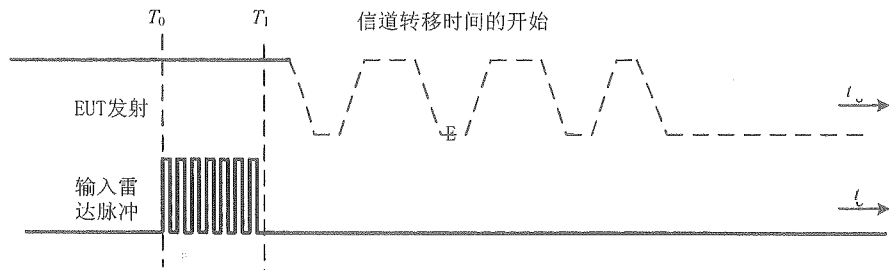
图7 在线监测期间进行雷达测试示例
