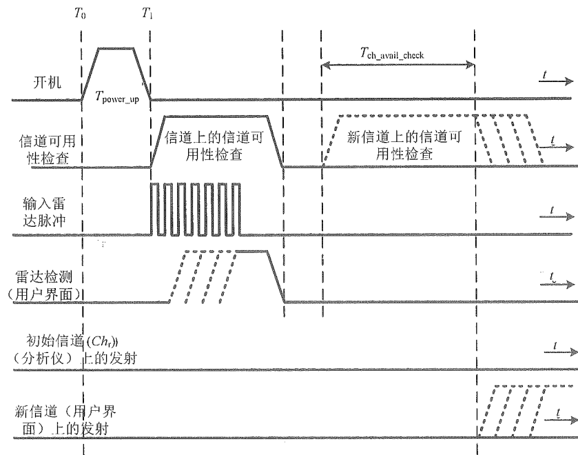
图4 在信道可用性检查时间开始进行雷达测试示例
